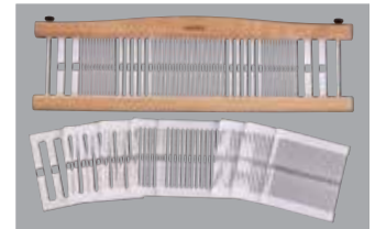
Peines de dientes variables
